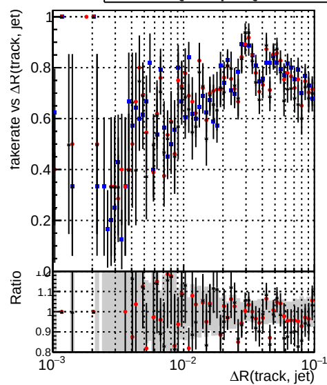
—●— DQMstep3_QCD_CKF —●— DQMstep3_QCD_default —●— DQMstep3_QCD_defaultNEWT
