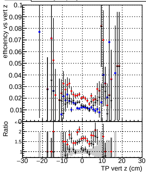
Efficiency vs vert z — DQMstep3_QCD_CKF — DQMstep3_QCD_default — DQMstep3_QCD_defaultNEWT
