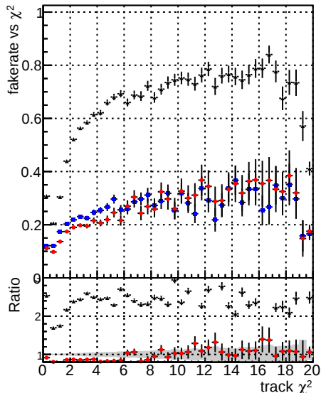
Fake rate vs. DOMstep3 OCB CKF DOMstep3 OCB default DOMstep3 OCB NEWT
