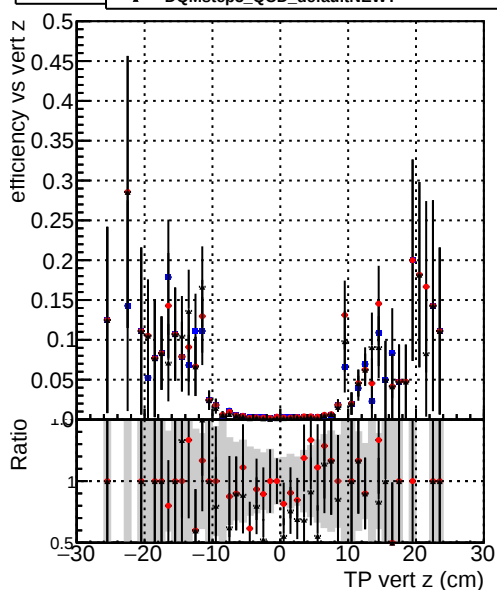
Efficiend —●— DQMstep3_QCD_default —★— DQMstep3_QCD_defaultNEWT
