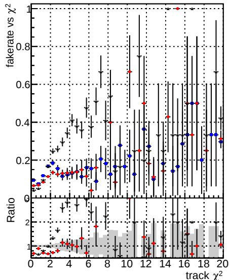
Fake rate vs. DOMstep3 OCB GKF DOMstep3 OCB default DOMstep3 OCB defaultNEWT
