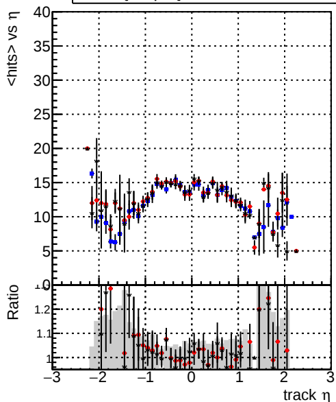
mean hit DQMstep3_QCD_CKF DQMstep3_QCD_default DQMstep3_QCD_defaultNEWT
