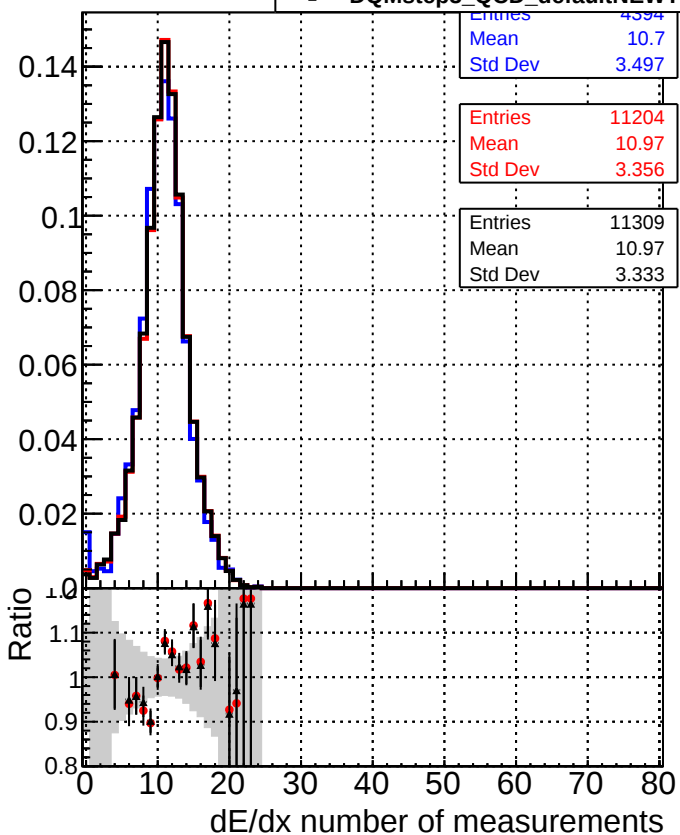
—■— DQMstep3_QCD_CKF —●— DQMstep3_QCD_default —*— DQMstep3_QCD_defaultNEWT
