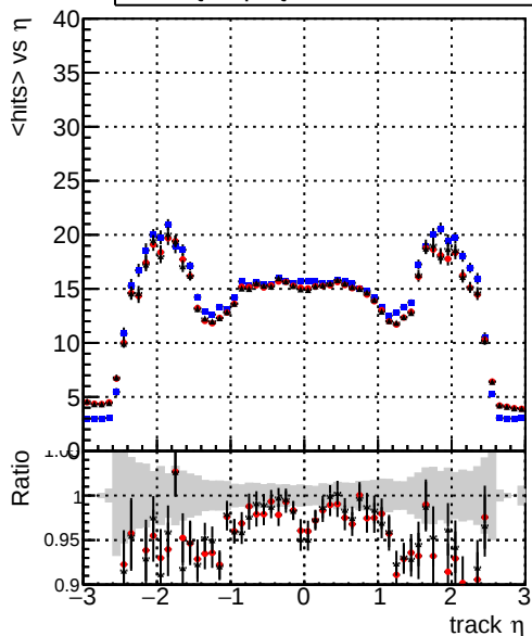
mean hits vs \eta — DQMstep3_QCD_CKF — DQMstep3_QCD_default — DQMstep3_QCD_defaultNEWT
