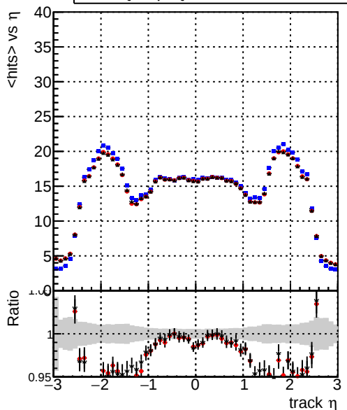
DQMstep3_QCD_CKF DQMstep3_QCD_default DQMstep3_QCD_defaultNEWT mean hits
