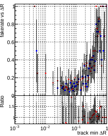
Fake rate vs \Delta R(\text{track, jet}) DOMstep3_QCD_CKF DOMstep3_QCD_default DOMstep3_QCD_defaultNEWT
