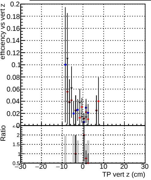
Efficiency vs TP vert z (cm) Legend: DQMstep3_QCD_ckpt DQMstep3_QCD_default DQMstep3_QCD_defaultNEWT
