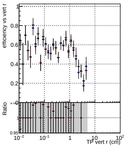
Efficiency vs vertpos Legend: DQMstep3_QCD_CKF DQMstep3_QCD_default DQMstep3_QCD_defaultNEWT
