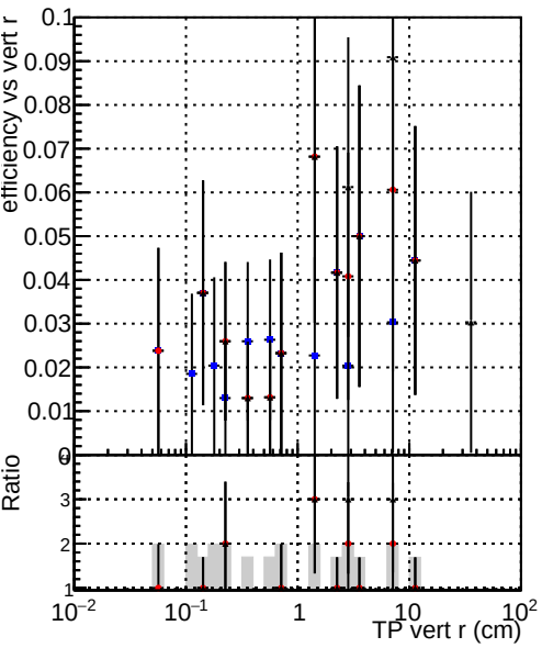
Efficiency vs TP vert r (cm) Legend: DQMstep3_QCD_CKF DQMstep3_QCD_default DQMstep3_QCD_defaultNEWT
