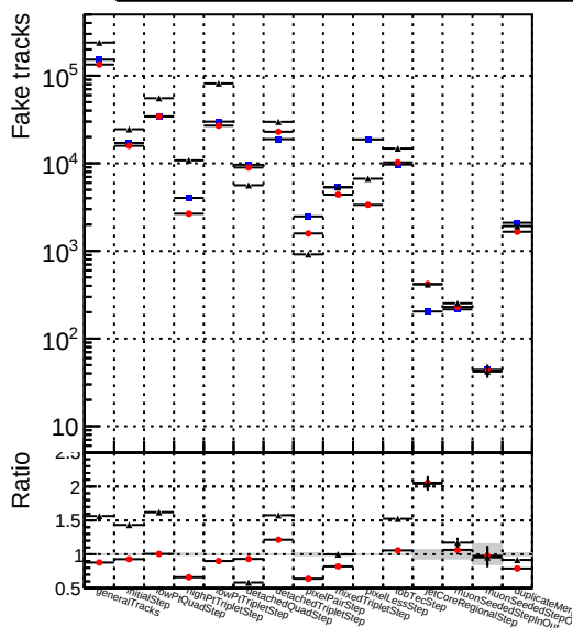
Number Legend —●— DQMstep3_QCD_default —★— DQMstep3_QCD_defaultNEWT
