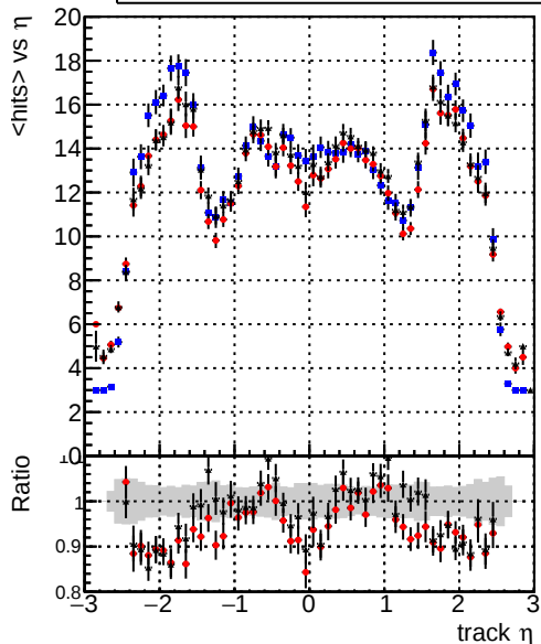
mean hits — DQMstep3_QCD_CKF — DQMstep3_QCD_default — DQMstep3_QCD_defaultNEWT
