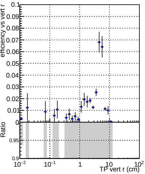
Efficiency vs TP vert r (cm) DQMstep3_QCD_defaultCHECK
