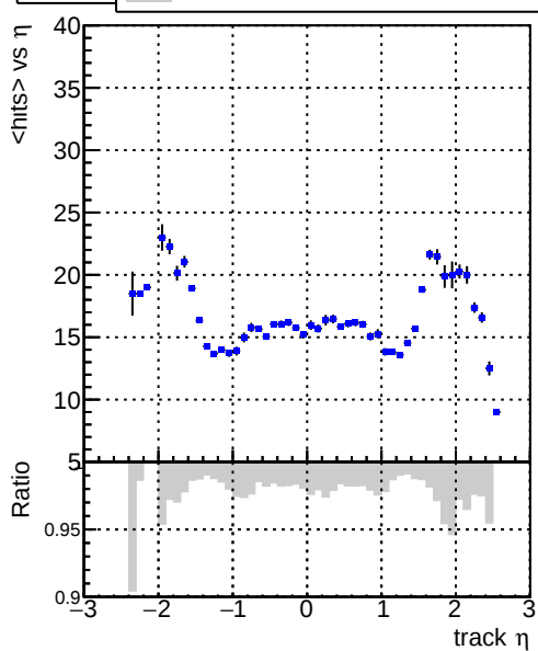
mean hit DQMstep3_QCD_defaultCHECK
