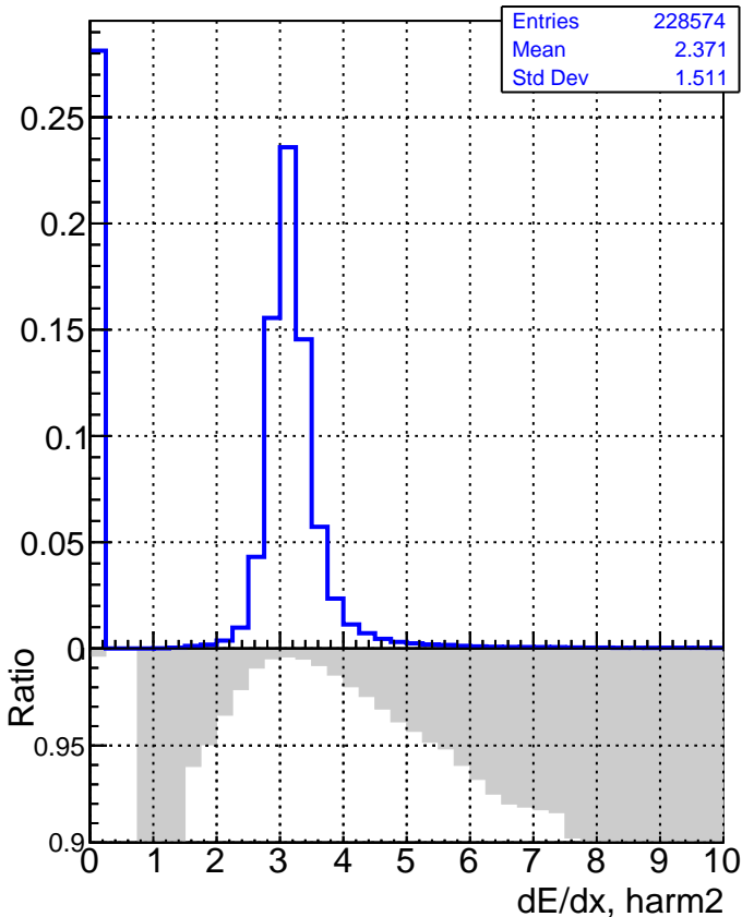
DQMstep3_QCD_defaultCHECK
