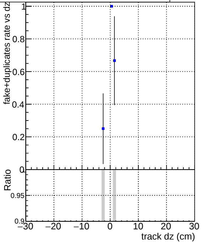
DQMstep3_QCD_defaultCHECK
