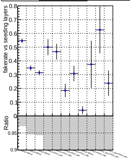
Fake rate vs. —●— DQMstep3_QCD_defaultCHECK
