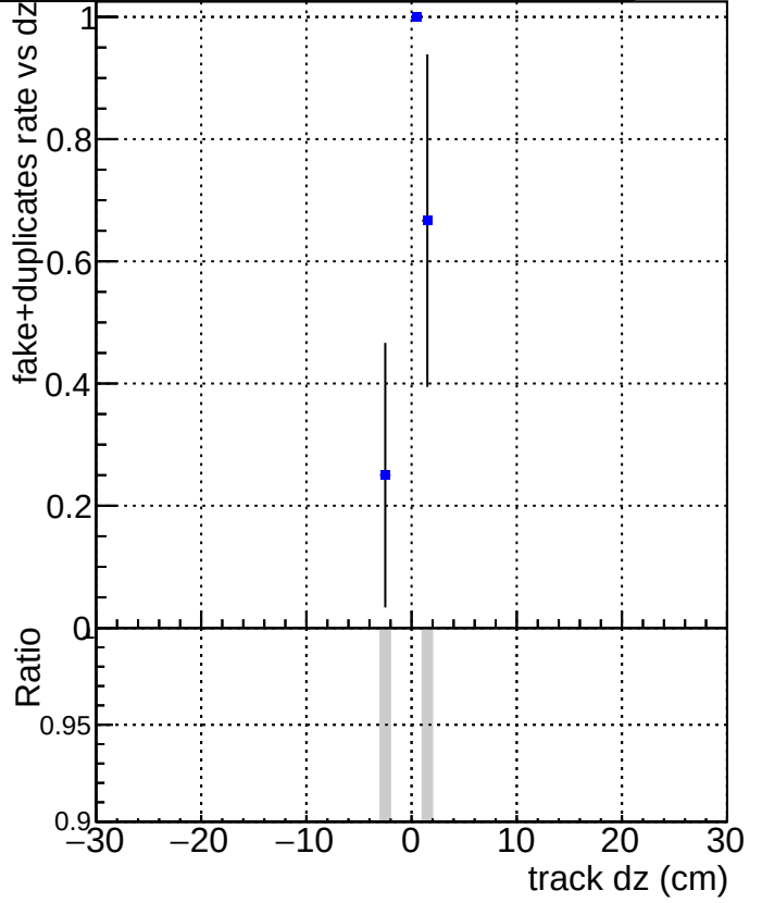
DQMstep3_QCD_defaultCHECK
