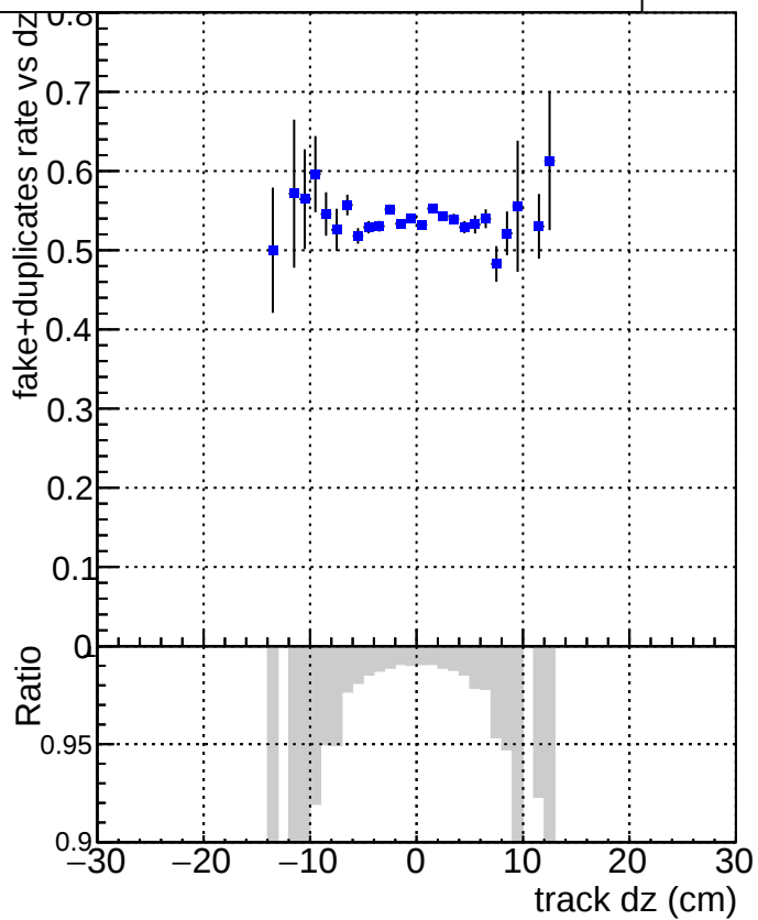
DQMstep3_QCD_defaultCHECK
