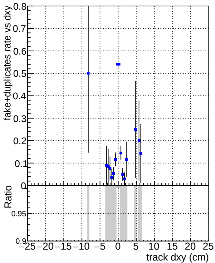
DQMstep3_QCD_defaultCHECK
