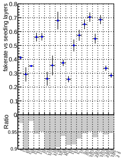
Fake rate vs. —●— DQMstep3_QCD_defaultCHECK
