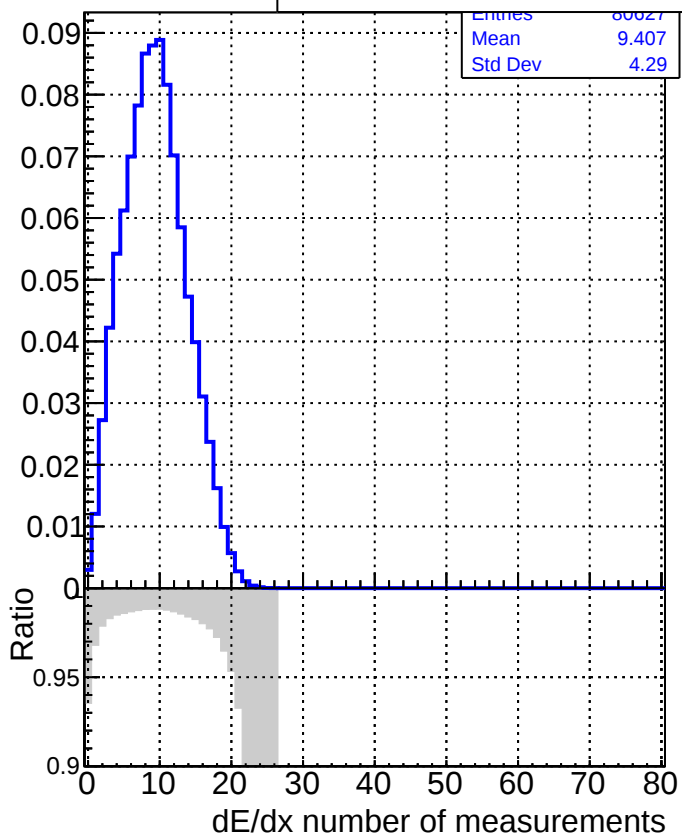
DQMstep3_QCD_defaultCHECK
