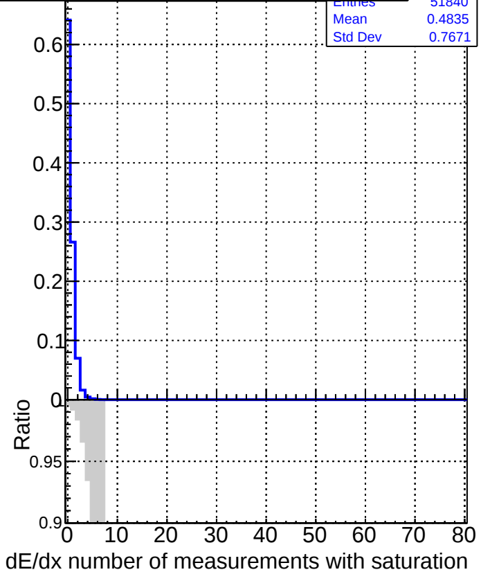
DQMstep3_QCD_defaultCHECK
