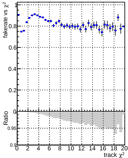
Fake rate vs. \chi^2 DQMstep3_QCD_defaultCHECK
