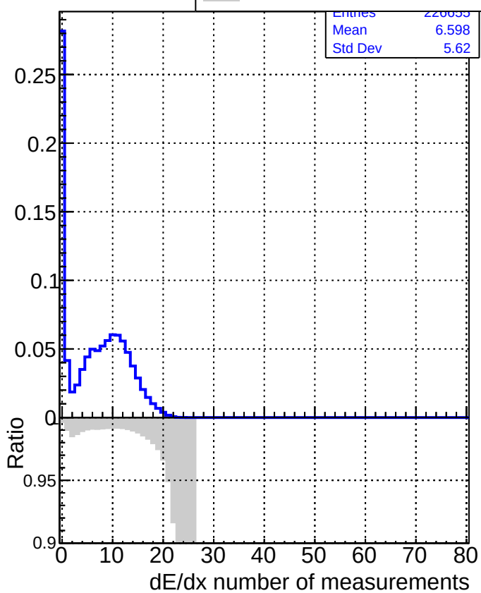
DQMstep3_QCD_defaultCHECK
