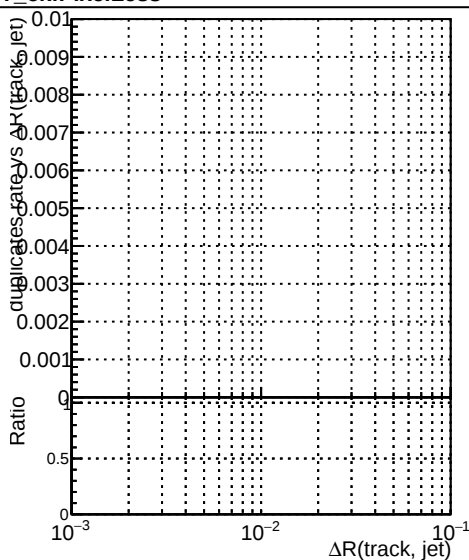
Legend: DQMstep3_DisplacedSUSY_CKF (blue circles) DQMstep3_DisplacedSUSY_default (red circles) DQMstep3_DisplacedSUSY_ckfPixelLess (black circles)
