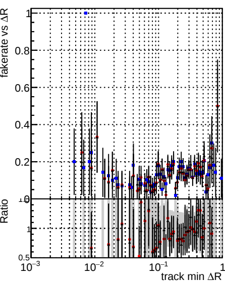
Fake rate vs \Delta R(\text{track, jet}) DQMstep3_DisplacedSUSY_CKF DQMstep3_DisplacedSUSY_default DQMstep3_DisplacedSUSY_ckfPixelLess
