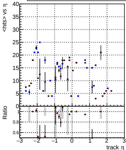
mean hits — DQMstep3_DisplacedSUSY_CKF — DQMstep3_DisplacedSUSY_default — DQMstep3_DisplacedSUSY_ckfPixelLess
