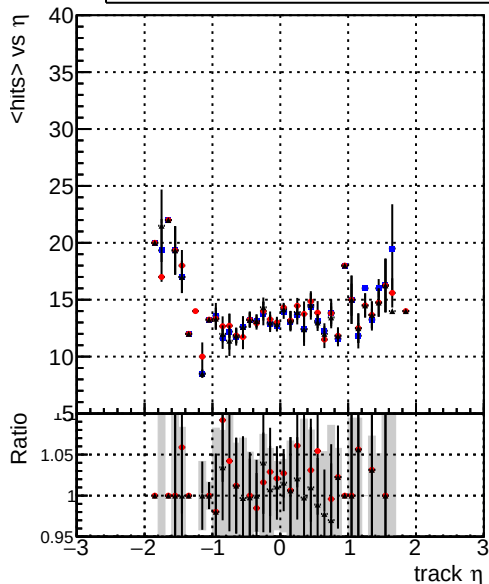
mean hit — DQMstep3_DisplacedSUSY_CKF — DQMstep3_DisplacedSUSY_default — DQMstep3_DisplacedSUSY_ckfPixelLess
