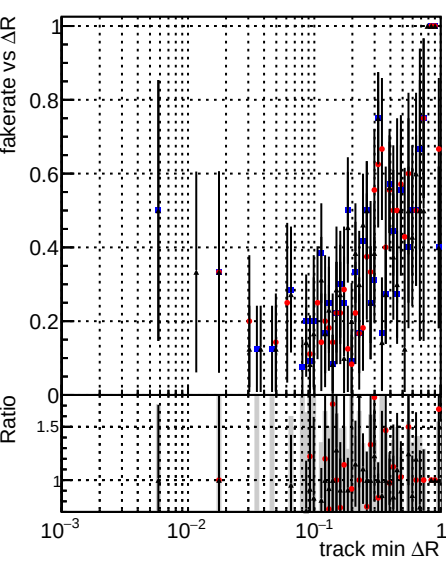
Fake rate vs \Delta R (track, jet) DQMstep3_DisplacedSUSY_CKF DQMstep3_DisplacedSUSY_default DQMstep3_DisplacedSUSY_ckfPixelLess
