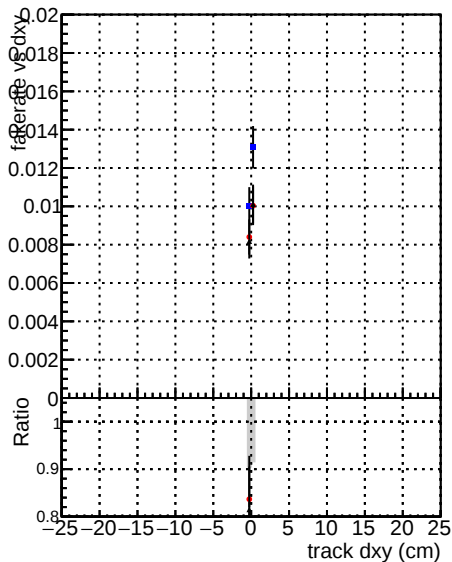
— DOMstep3 DisplacedSUSY CKF — DOMstep3 DisplacedSUSY default — DOMstep3 DisplacedSUSY-ckfPixelLess
