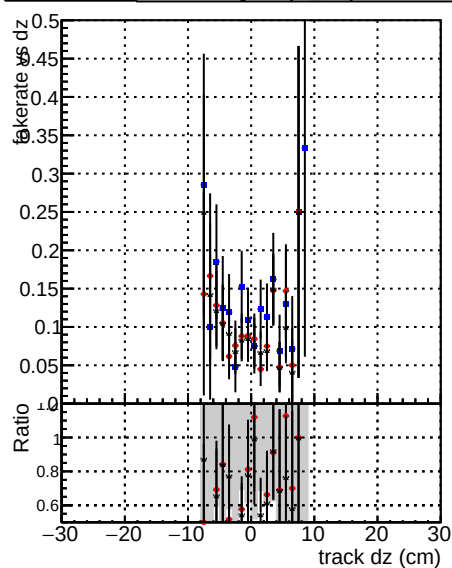
Fake rate vs dz —•— DOMstep3 DisplacedSUSY CKF —•— DOMstep3 DisplacedSUSY default —•— DOMstep3 DisplacedSUSY ckfPixelLess
