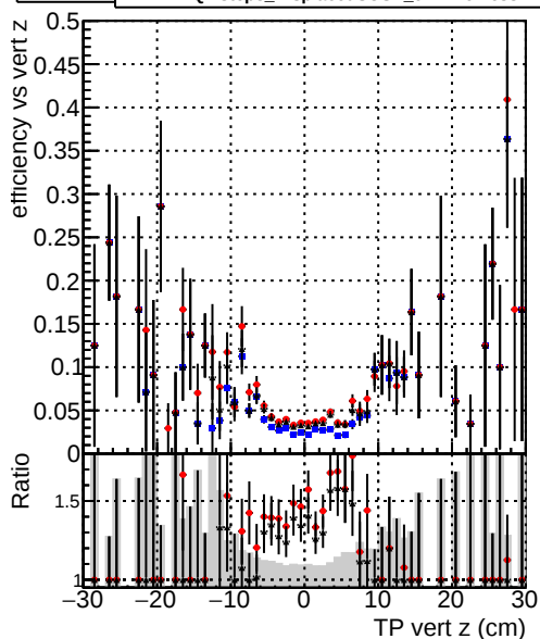
Efficiency vs vert z —●— DQMstep3_DisplacedSUSY_CKF —●— DQMstep3_DisplacedSUSY_default —●— DQMstep3_DisplacedSUSY_ckptPixelLess
