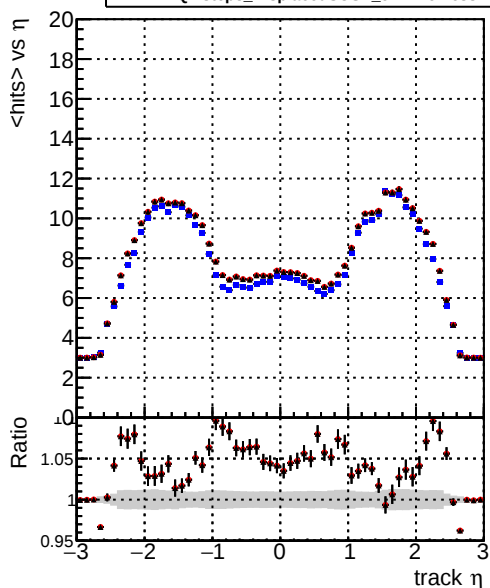
mean hits — DQMstep3_DisplacedSUSY_CKF — DQMstep3_DisplacedSUSY_default — DQMstep3_DisplacedSUSY_ckfPixelLess
