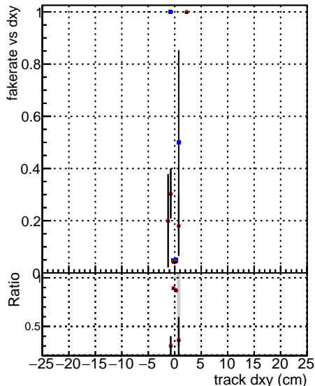
—●— DQMstep3 DisplacedSUSY CKF —●— DQMstep3 DisplacedSUSY default —●— DQMstep3 DisplacedSUSY CKF PixelLess
