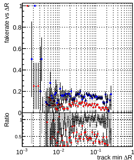
—●— DQMstep3_DisplacedSUSY_CKF —●— DQMstep3_DisplacedSUSY_default —●— DQMstep3_DisplacedSUSY_ckfPixelLess
