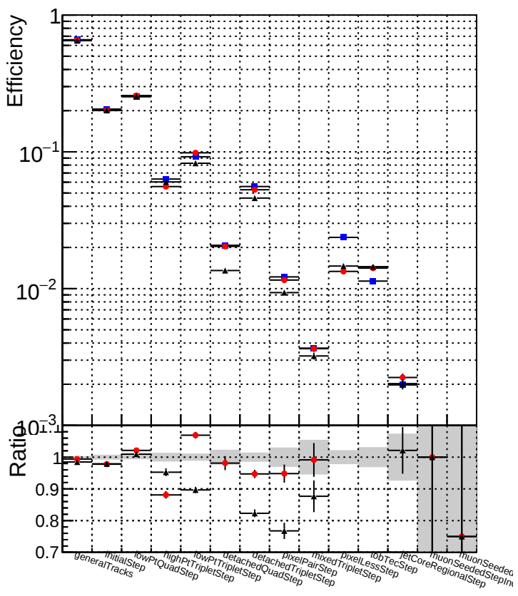
DQMstep3_DisplacedSUSY_CKF DQMstep3_DisplacedSUSY_default DQMstep3_DisplacedSUSY_defaultNEWT
