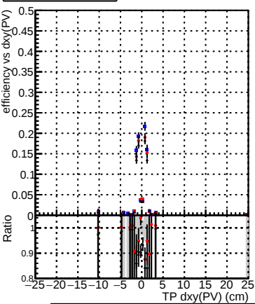
Efficiency vs Dxy(PV) Legend: DQMstep3_DisplacedSUSY_CKF DQMstep3_DisplacedSUSY_default DQMstep3_DisplacedSUSY_defaultNEWT
