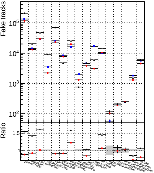
Number Legend —●— DQMstep3_DisplacedSUSY_default —★— DQMstep3_DisplacedSUSY_defaultNEWT
