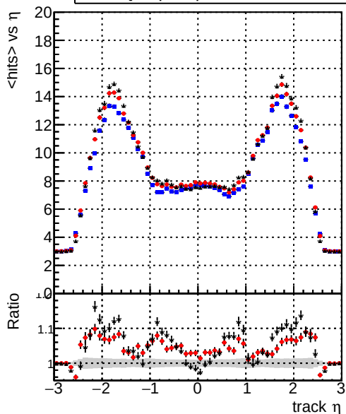
mean hit — DQMstep3_DisplacedSUSY_CKF — DQMstep3_DisplacedSUSY_default — DQMstep3_DisplacedSUSY_defaultNEWT
