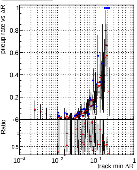
—•— DQMstep3_DisplacedSUSY_CKF —•— DQMstep3_DisplacedSUSY_default —•— DQMstep3_DisplacedSUSY_defaultNEWT
