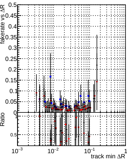
—•— DQMstep3_DisplacedSUSY_CKF —•— DQMstep3_DisplacedSUSY_default —•— DQMstep3_DisplacedSUSY_defaultNEWT
