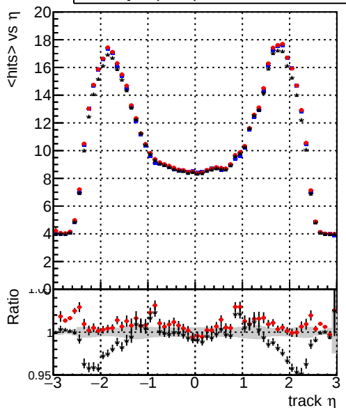
mean hit — DQMstep3_DisplacedSUSY_CKF — DQMstep3_DisplacedSUSY_default — DQMstep3_DisplacedSUSY_defaultNEWT
