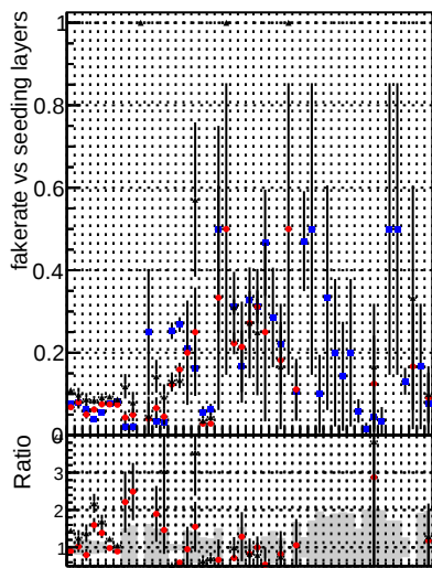
Fake rate vs. DOMstep3 DisplacedSUSY CKF DOMstep3 DisplacedSUSY default DOMstep3 DisplacedSUSY default NEWT
