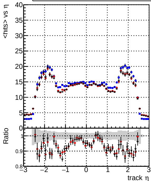
DQMstep3_DisplacedSUSY_CKF DQMstep3_DisplacedSUSY_default DQMstep3_DisplacedSUSY_defaultNEWT mean hits
