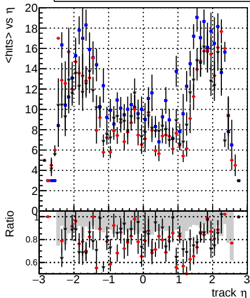
— DQMstep3_DisplacedSUSY_CKF — DQMstep3_DisplacedSUSY_default — DQMstep3_DisplacedSUSY_defaultNEWT mean hit
