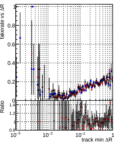
Legend: DQMstep3_DisplacedSUSY_CKF (blue circles), DQMstep3_DisplacedSUSY_default (red circles), DQMstep3_DisplacedSUSY_defaultNEWT (black circles)
