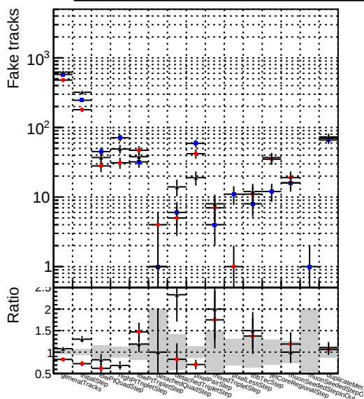
Number Legend ● DQMstep3_DisplacedSUSY_default ▲ DQMstep3_DisplacedSUSY_defaultNEWT
