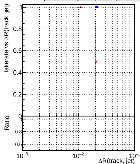
—●— DQMstep3_DisplacedSUSY_CKF —●— DQMstep3_DisplacedSUSY_default —●— DQMstep3_DisplacedSUSY_NEWT
